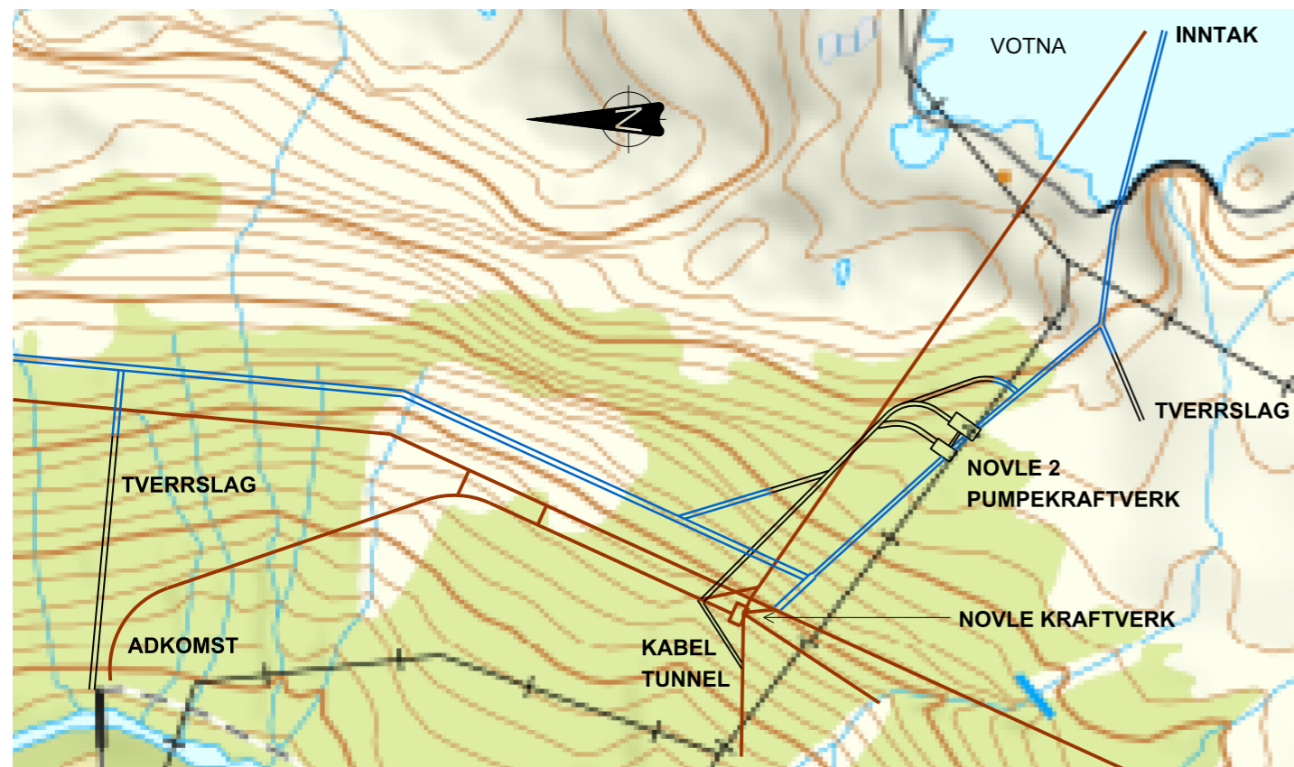
PLAN KRAFTSTASJONSOMRÅDE
